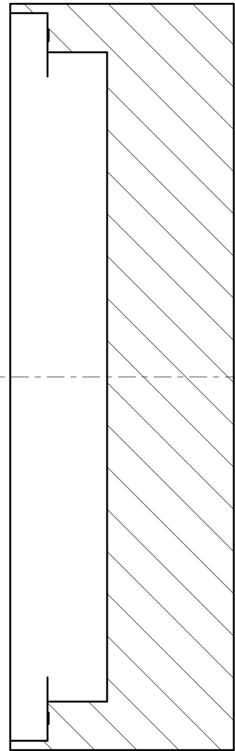
Fräsbild Flügel
