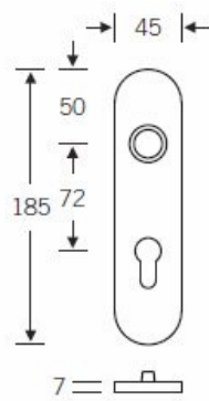
Provedení se štítkem
