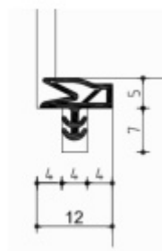
Dvevní těsnění Deventer pro bezfalcové dveře
